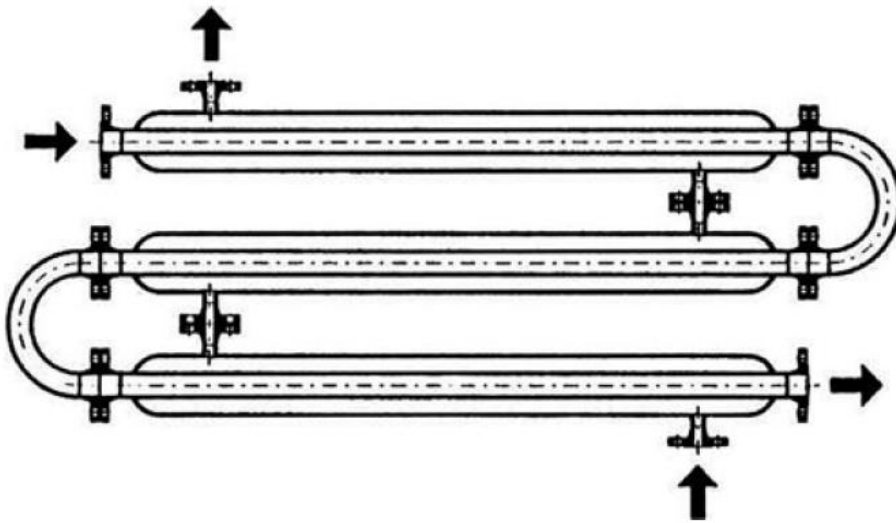
Wymiennik typu rura w rurze, trójsekcyjny.
