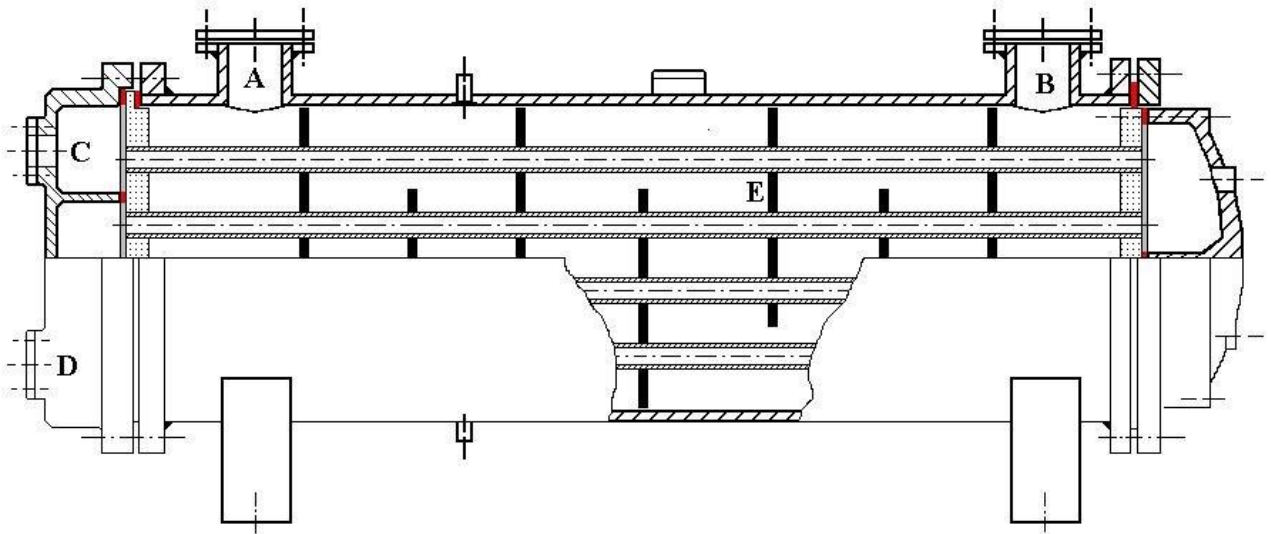
Wymiennik płaszczowo-rurowy, czterodrogowy, z przegrodami segmentowymi. W kolorze czerwonym przedstawiono uszczelnienia.
