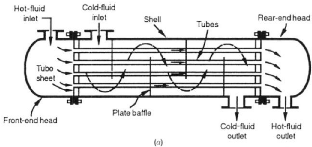
Wymiennik ciepła płaszczowo rurowy, jednoprzepływowy, współprądowy, z przegrodami segmentowymi.
